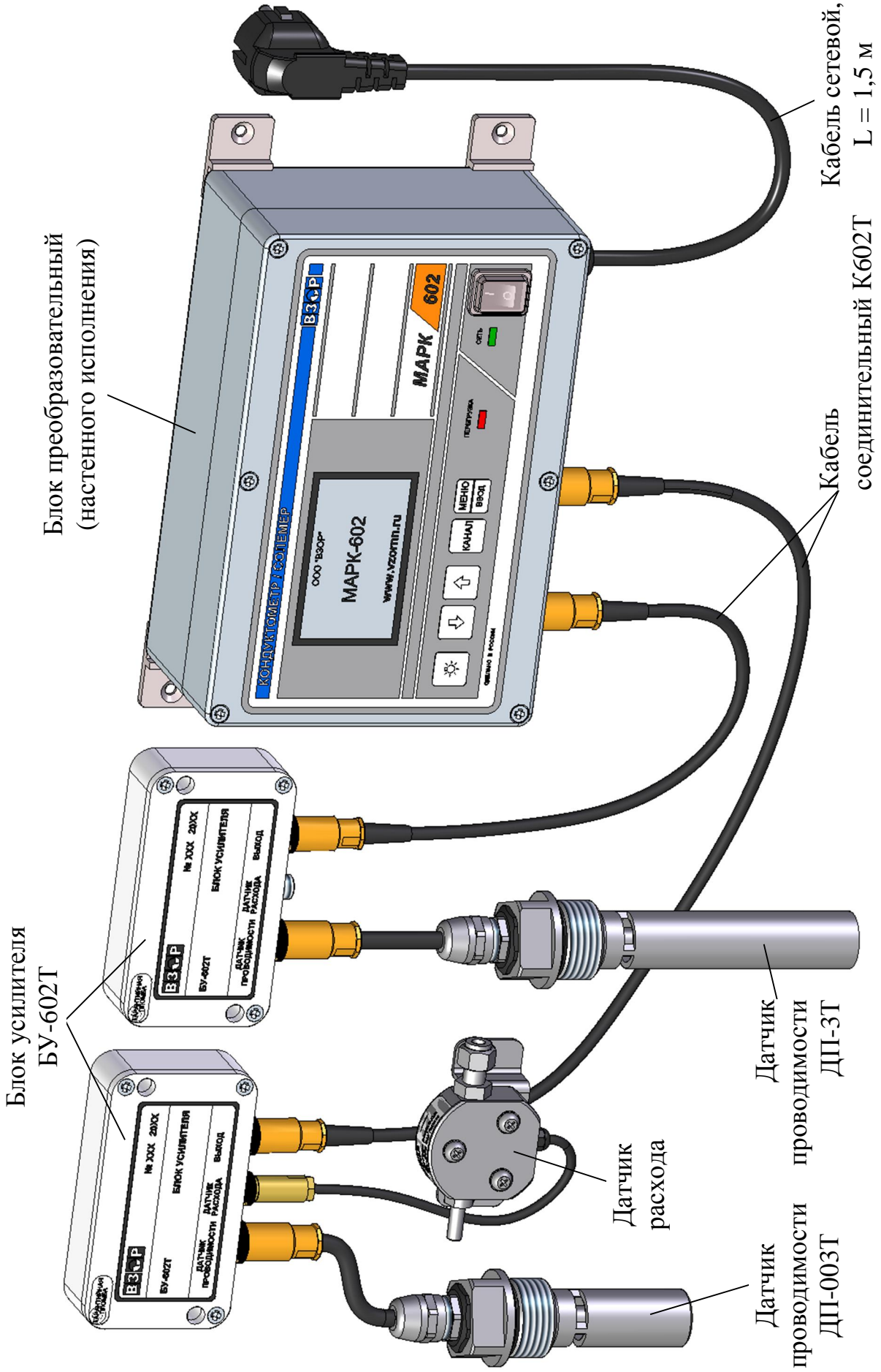
Рисунок 1.1 – Кондуктометр-солемер MARK-602T/1
